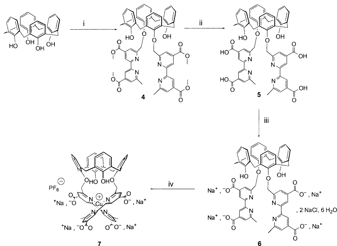
Scheme 1. i) 3 , MeCN, \text{K}_2\text{CO}_3 , reflux, 83%; ii) a) NaOH, \text{H}_2\text{O} , EtOH, reflux; b) HCl, pH 3–4, 80%; iii) NaOH, \text{H}_2\text{O} , pH 7, 100%; iv) \text{Cu}(\text{MeCN})_4\text{PF}_6 , MeCN, \text{H}_2\text{O}
